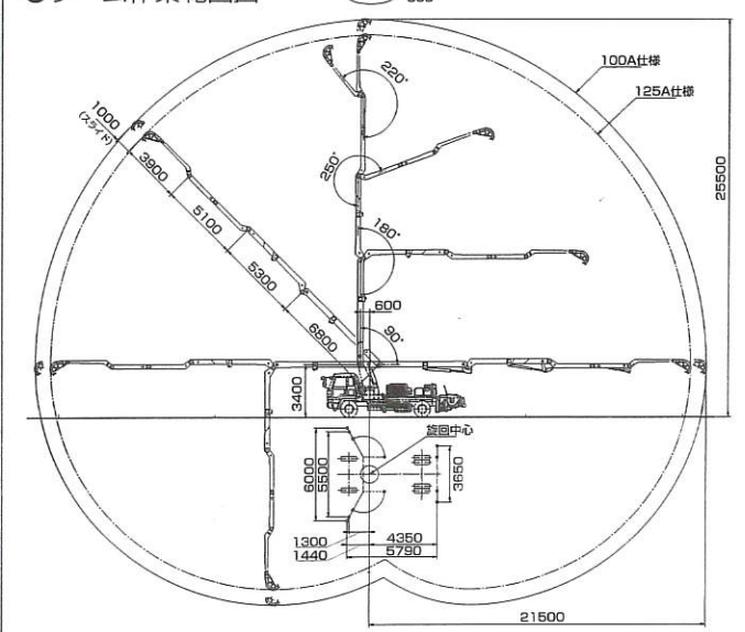
●ブーム作業範囲図
