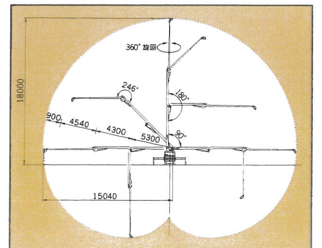
■ブーム作業範囲図 (単位:mm)
