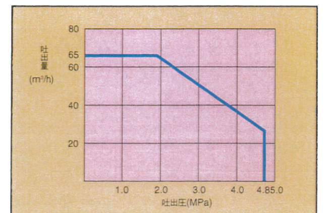
■性能曲線
