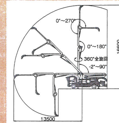
■ブーム作業範囲図(単位:mm)
