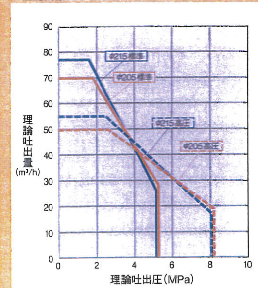
■性能曲線
