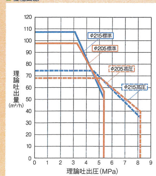
■性能曲線
