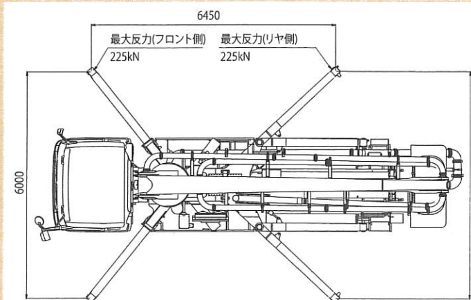
■アウトリガ張幅及び反力
